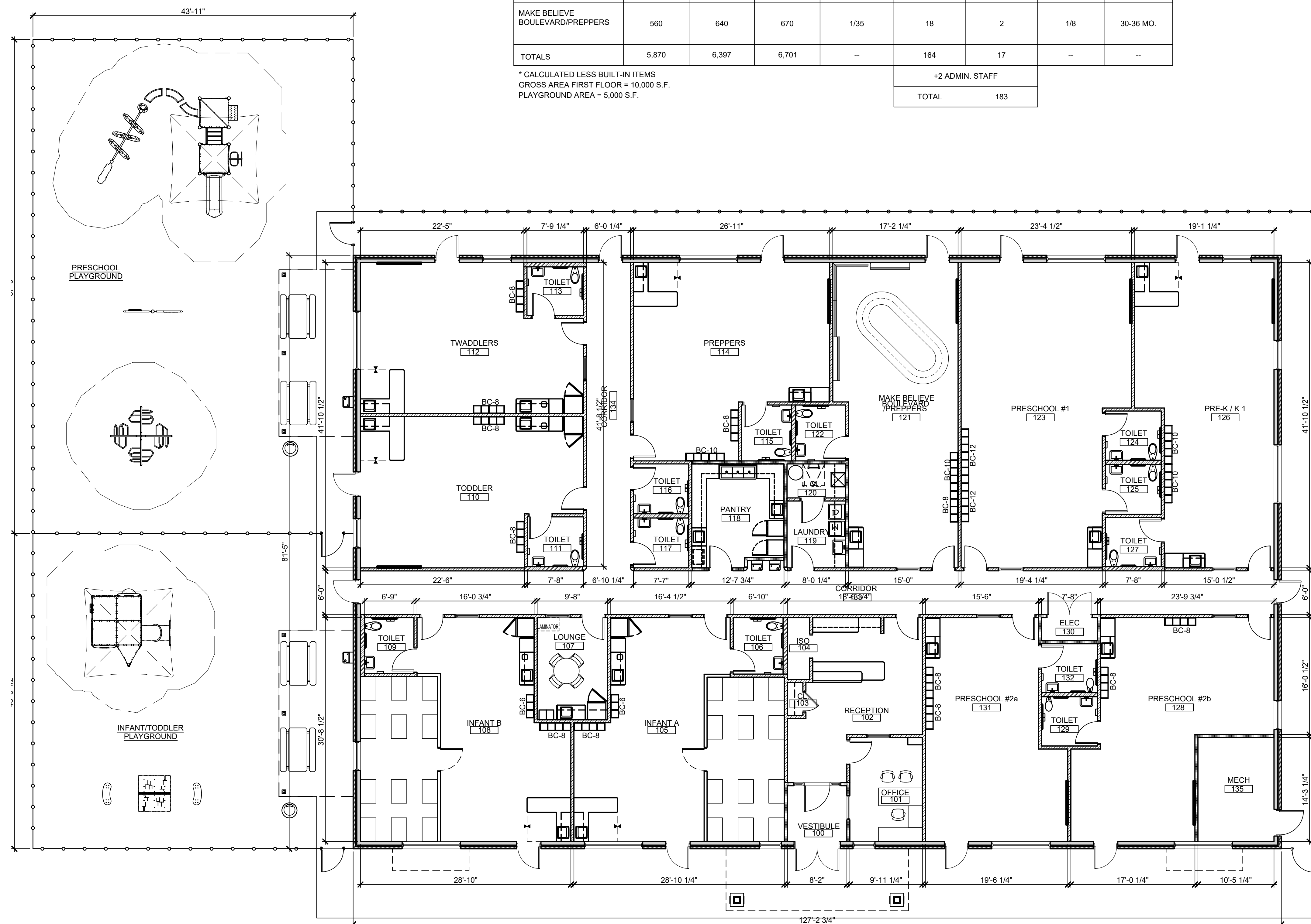
1 LICENSING PLAN scale: 1/8"=1'-0"
